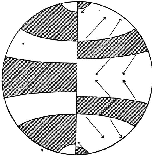
वर्षा वर्षा के क्षेत्र चिह्नित हैं दाब उच्च दाब के क्षेत्र चिह्नित हैं चित्र ४०—वर्षा और दाब का सम्बन्ध
